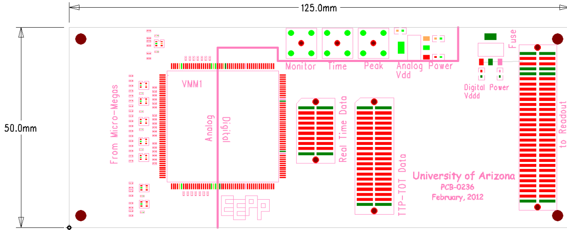
LAYER: TOP
