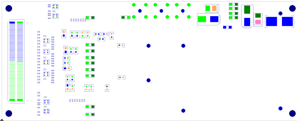
LAYER: Bottom
