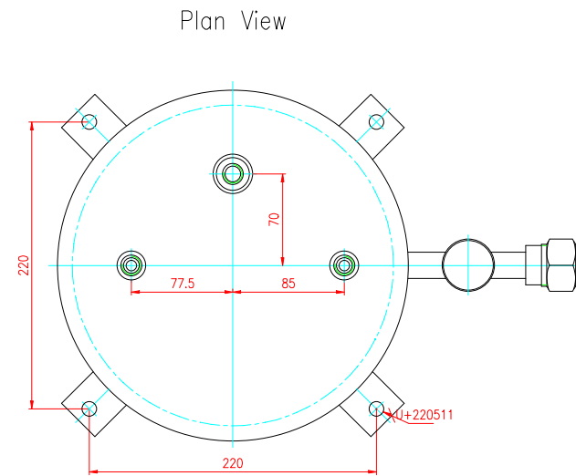
Fig.7 Cryostat.
